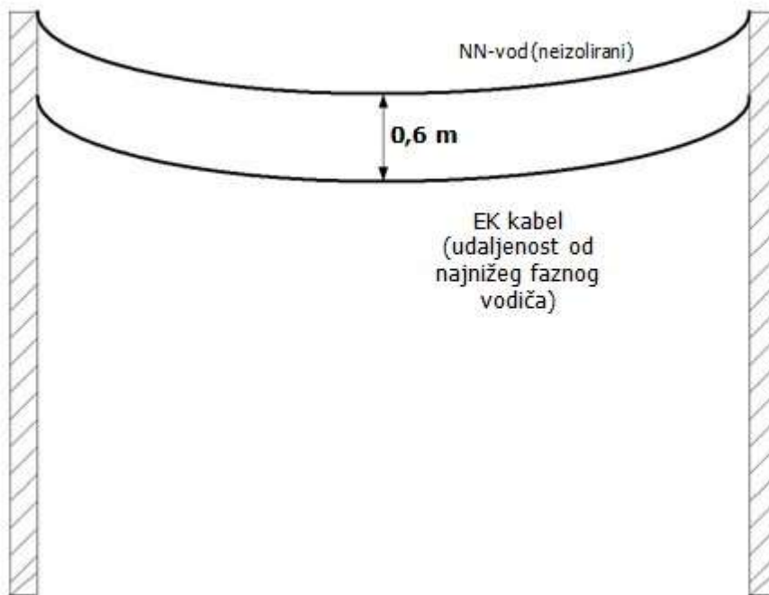
Slika 3 Razmak između EK kabela i NN neizoliranog voda u sredini raspona
