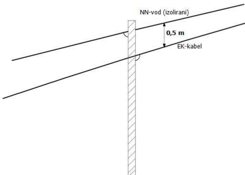
Slika 2 Razmak između EK kabla i NN izoliranog voda na stupu
