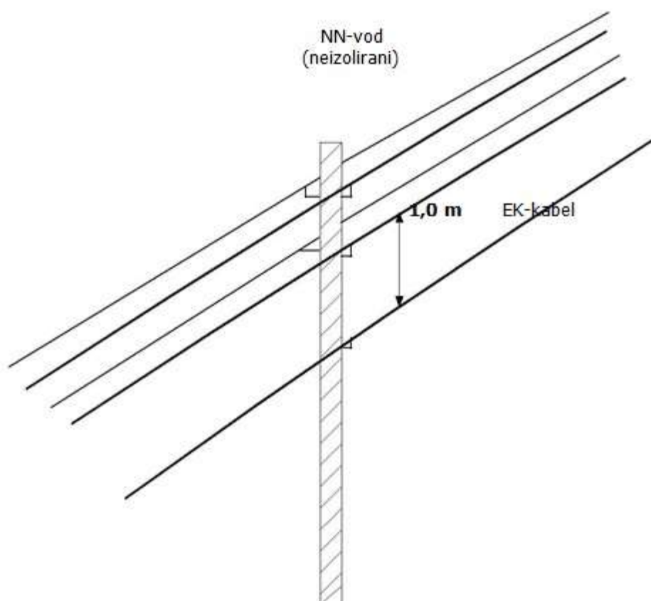
Slika 1 Razmak između EK kabla i NN neizoliranog voda na stupu
